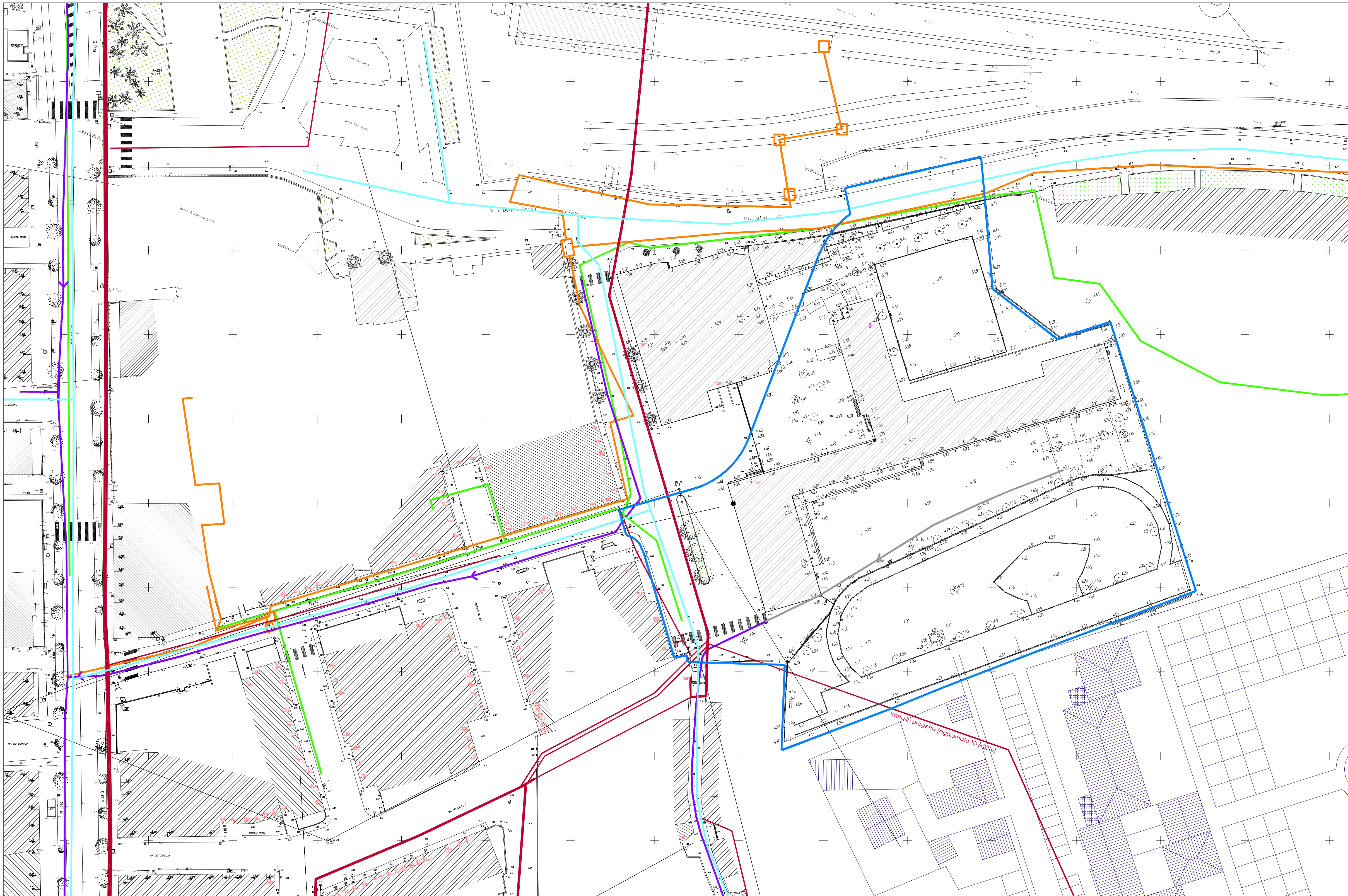
STATO DI FATTO SERVIZI A RETE - scala 1:500
