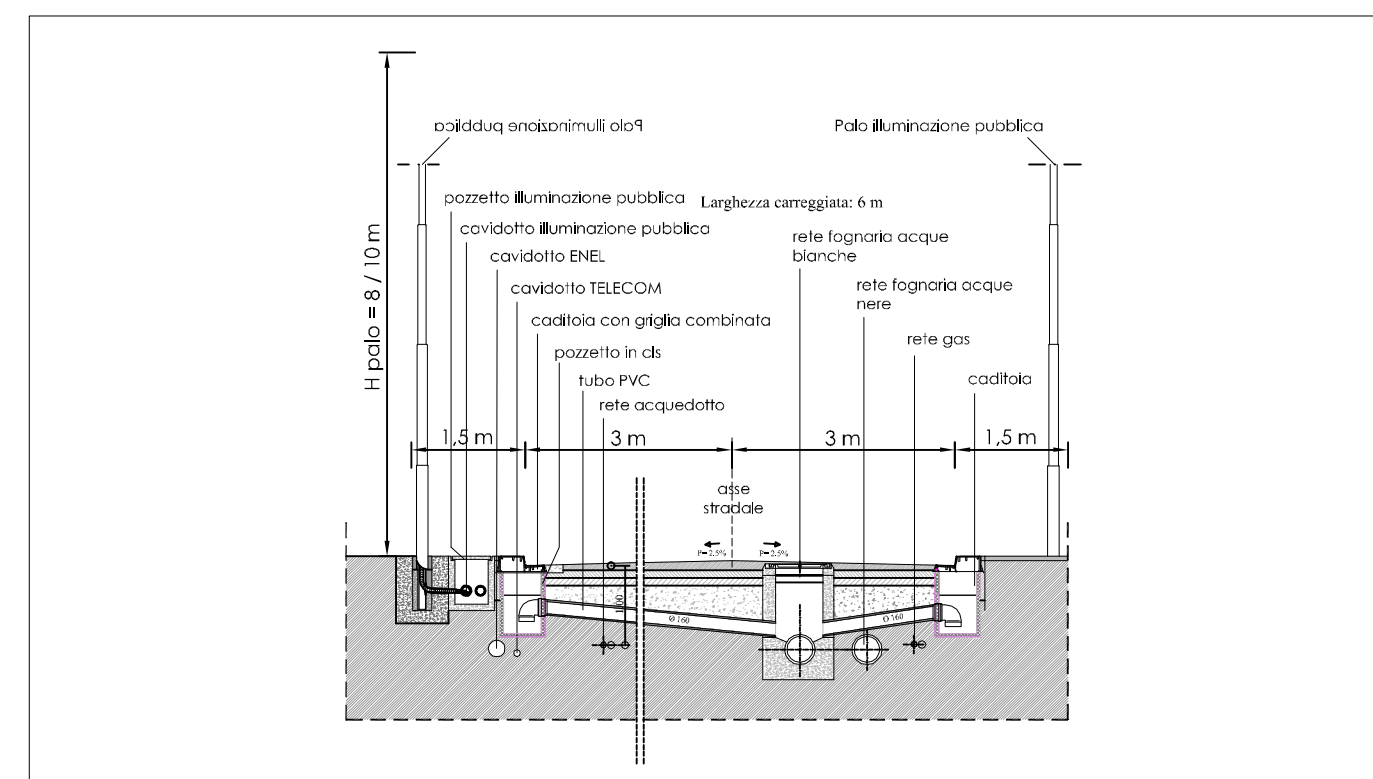
SEZIONE "A": sezione stradale tipo - scala 1:100
