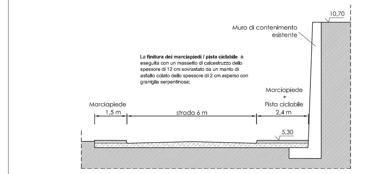
SEZIONE "B": sezione strada e pista ciclabile - scala 1:100
