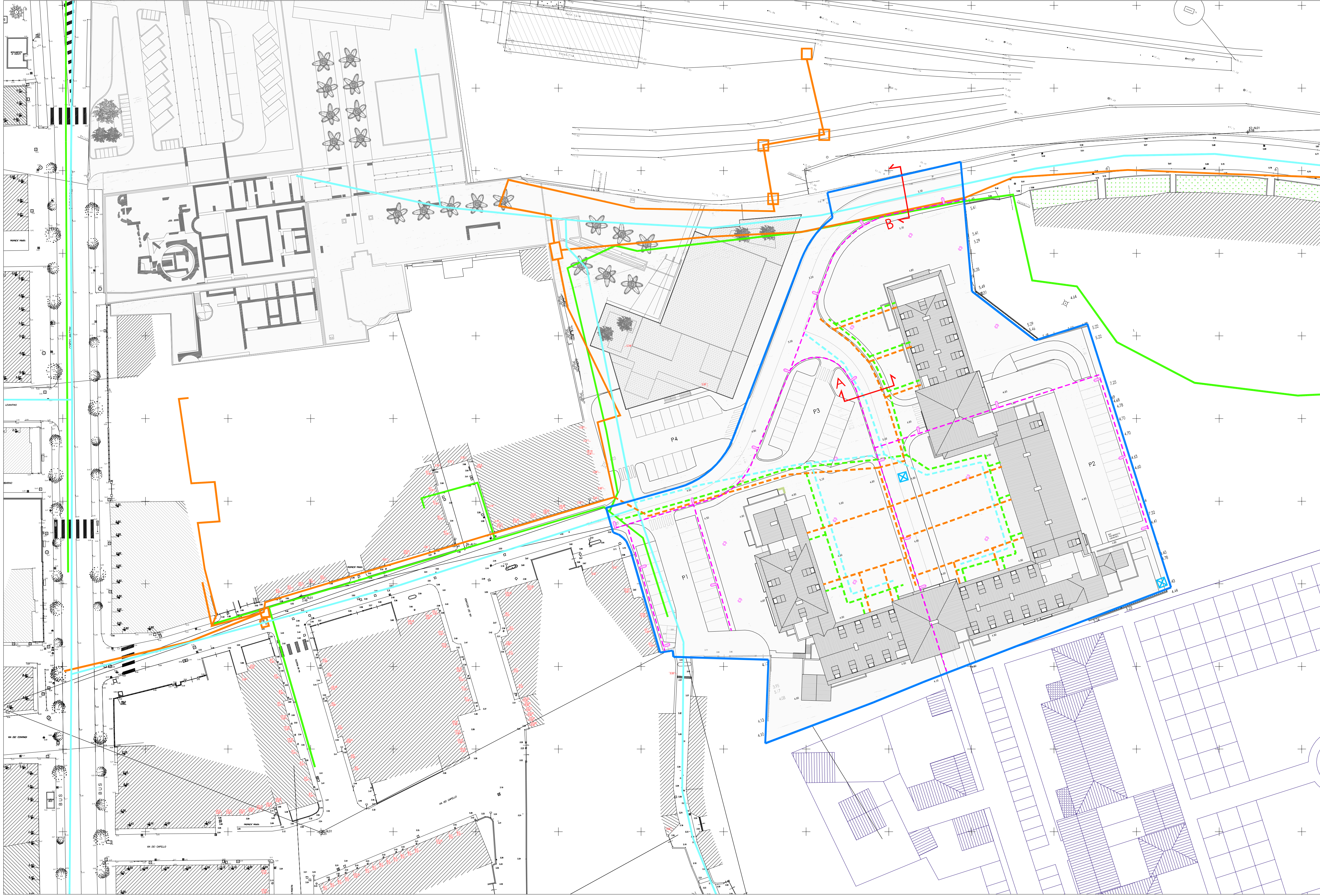
STATO DI PROGETTO SERVIZI A RETE - scala 1:500
