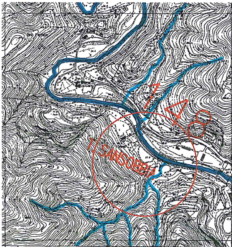
Estratto cartografico Piano di Bacino "Torrente Sansobbia" - Carta della Suscettività al dissesto, scala 1:10000
