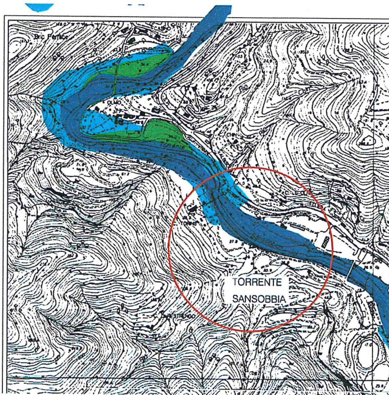
Estratto cartografico Piano di Bacino "Torrente Sansobbia" - Carta degli Interventi, scala 1:10000 Area d'intervento
